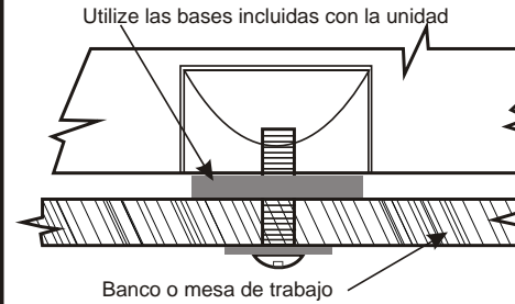
FIGURA 11. Fije el Dispensador al extremo superior de la mesa o banco de trabajo.
