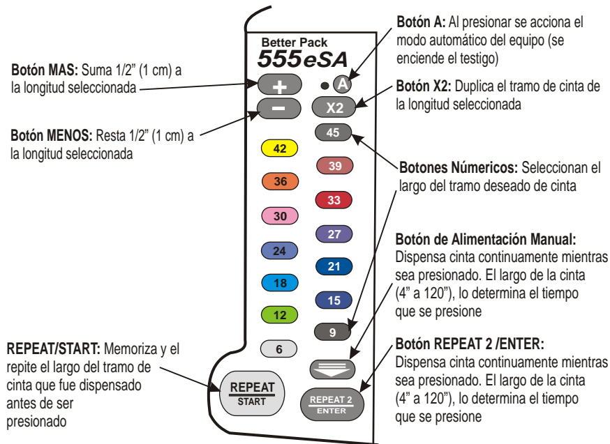
FIGURA 16 b. Panel de Control para Selección de Largo de Cinta
