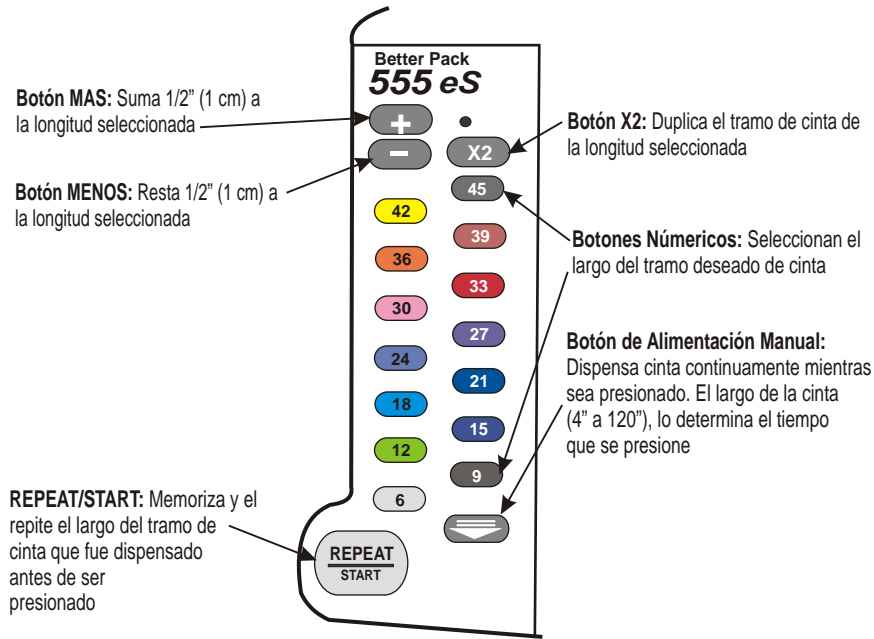
FIGURA 16 a. Panel de Control para Selección de Largo de Cinta
